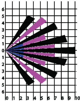
Erfassungsbereich Draufsicht
