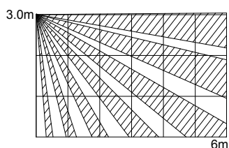
Erfassungsbereich Seitenansicht
